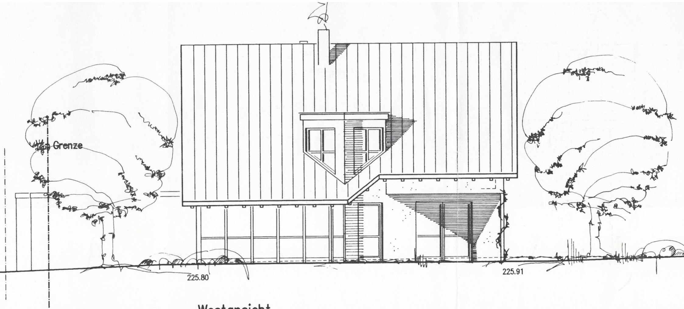
Westansicht
